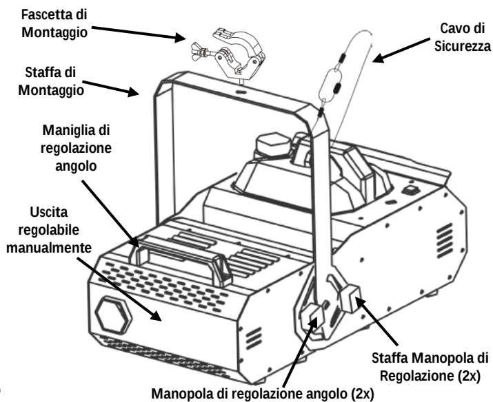
Schema di Montaggio dell'Unità
