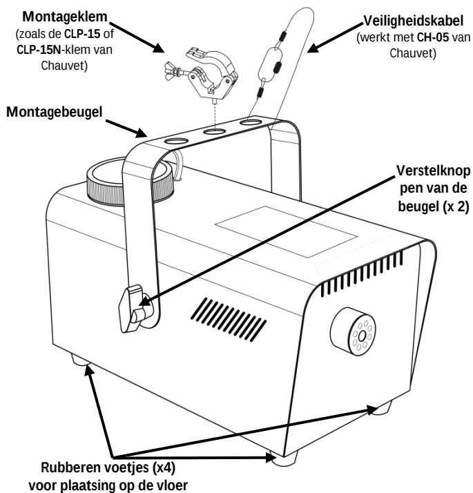
Montagediagram
