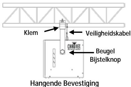
Hangende Bevestiging
