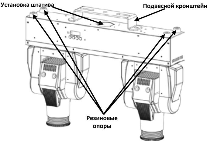
Схема монтажа устройства
