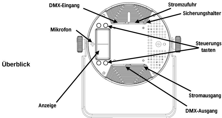
Ansicht des Rückwärtigen Bedienfelds
