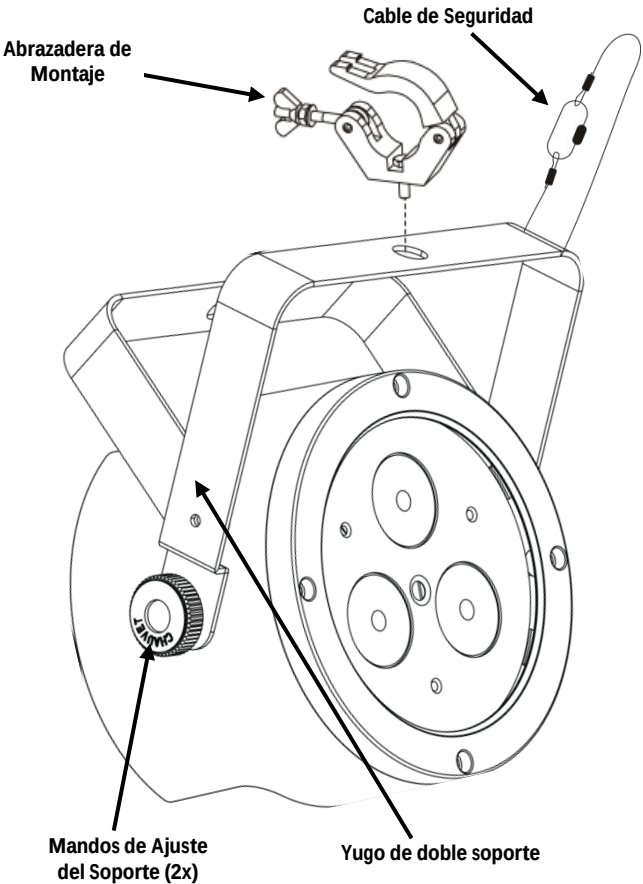
Diagrama de Montaje
