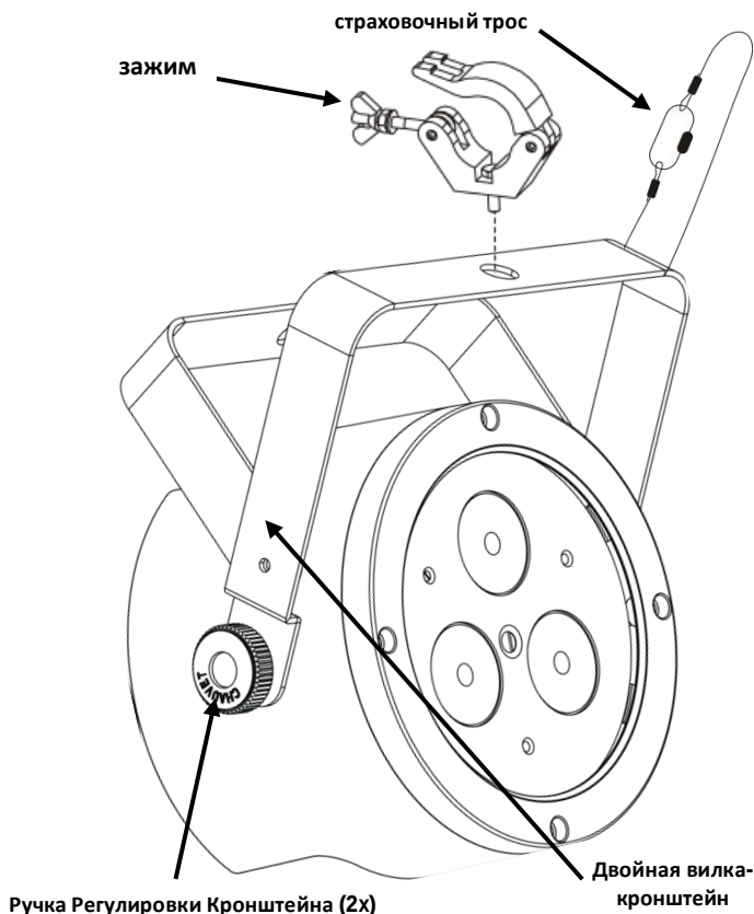
Схема монтажа
