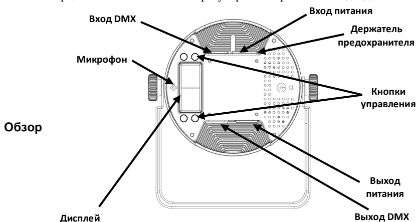
Вид задней панели
